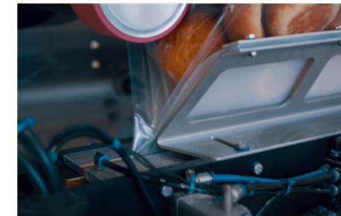
④ Schrägschweißung
