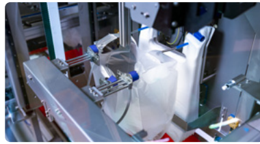
2 Beutel öffnen
